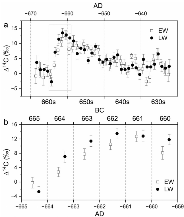
Fig. 2 - A sub-annually sampled ^{14}\text{C} archive from tree rings of Japanese cedar ( Cryptomeria japonica ). Earlywood (EW) and latewood (LW) ^{14}\text{C} concentrations of each annual ring are presented a) for 669-633 BC period and b) detailed for 665-660 BC period. The BC and AD years represent the timelines A and F, respectively (see Fig. 1). The ^{14}\text{C} data originate from Sakurai et al. (2020). / Un archivio di ^{14}\text{C} campionato con risoluzione sub-annuale dagli anelli di crescita di cedro giapponese Cryptomeria japonica (Thunb. ex L.f.) D.Don. Le concentrazioni di ^{14}\text{C} del legno precoce (EW) e del legno tardivo (LW) di ciascun anello annuale sono presentate: a) per il periodo 669-633 a.C., e b) in dettaglio per il periodo 665-660 a.C. Gli anni a.C. e d.C. rappresentano rispettivamente le cronologie A e F (vedi Fig. 1). I dati del ^{14}\text{C} provengono da Sakurai et al. (2020).
