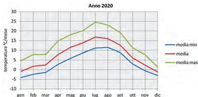
Fig. 5 - Temperature medie mensili nel 2020. / Average monthly temperatures in 2020.
